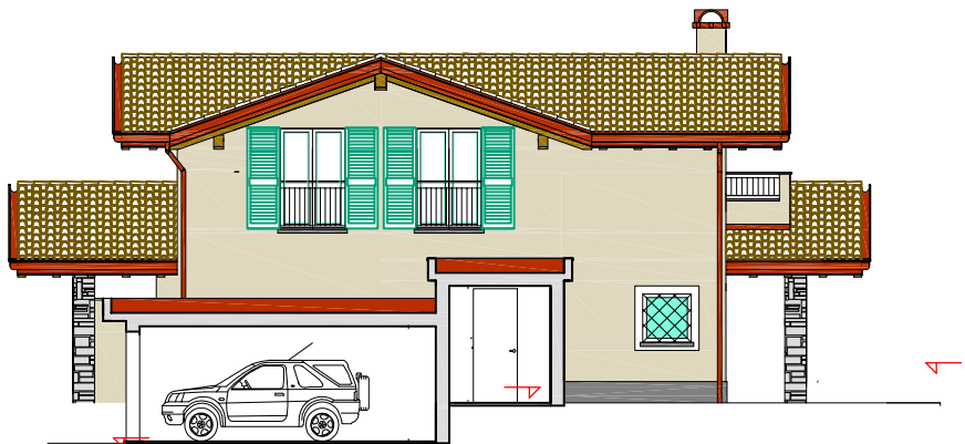
prospetto nord / sezione autorimessa - unità abitativa C
